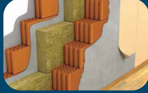
Ortak Duvar Ses Yalıtımı
